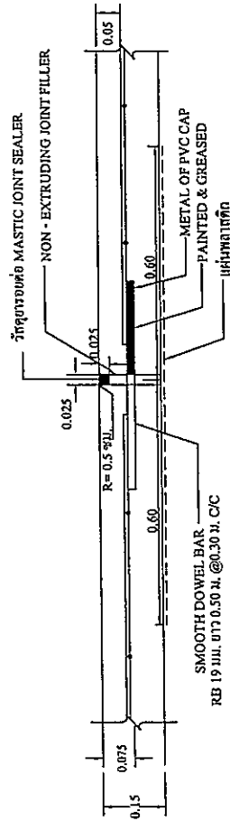
ขยายรอยต่อ ② expansion joint ทุกระยะไม่เกิน 100 เมตร
