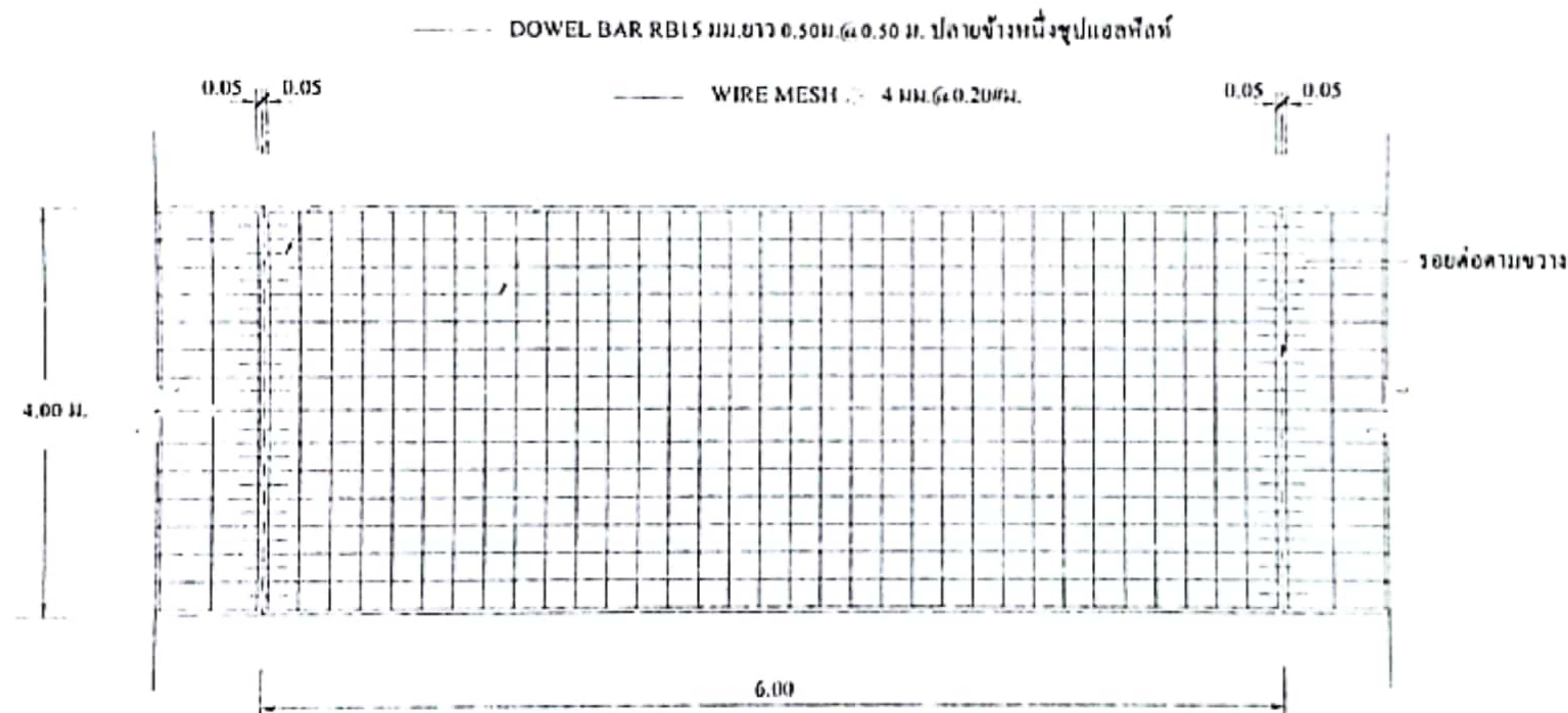
แบบแปลนการวางเหล็กตะแกรง
