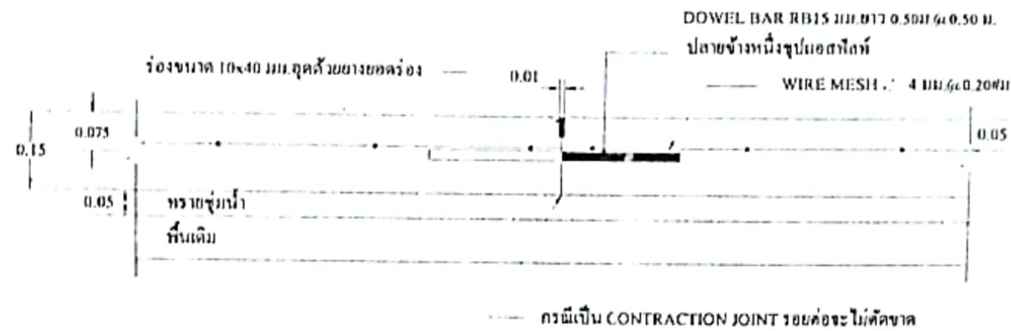
ขยายรอยต่อ 1 contraction joint ทุกระยะ 6 เมตร
