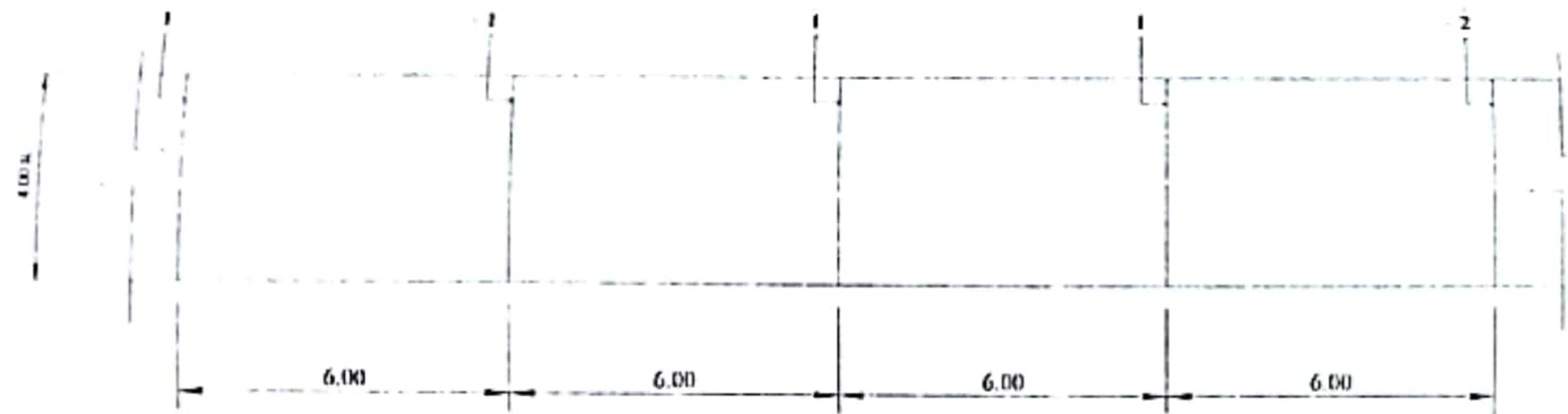
แบบแปลนถนนคอนกรีตเสริมเหล็ก
